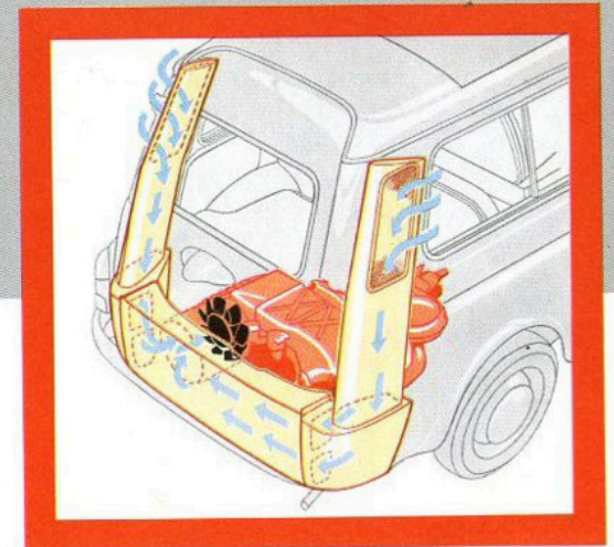
De circulatie van de koellucht
